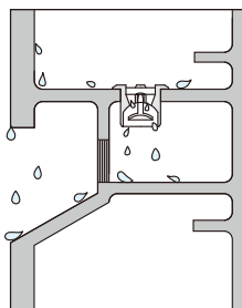
逆流防止弁及び取付図
