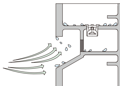
逆流防止機構
